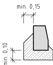
SILNIČNÍ OBRUBNÍK 150/250
