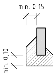
CHODNÍKOVÝ OBRUBNÍK 80/250
