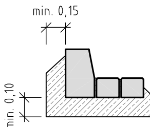
SILNIČNÍ OBRUBNÍK 150/250 S DVOŘÁDKEM ZE ŽULOVÉ KOSTKY
