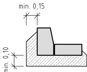
SILNIČNÍ OBRUBNÍK 150/250 S PŘÍDLAŽBOVOU DLAŽDICÍ
