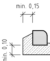
SILNIČNÍ OBRUBNÍK 150/150 - NÁJEZDOVÝ
